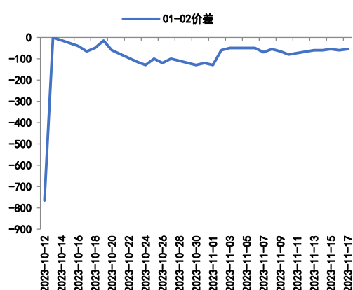
图6：工业硅期货合约S2401—S2402价差
