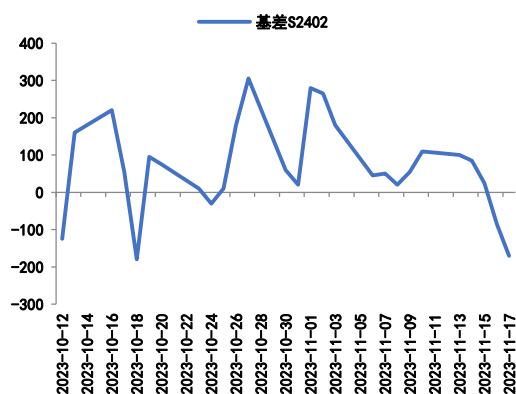
图4：工业硅期货合约S2402基差
