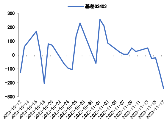
图5：工业硅期货合约S2403基差
