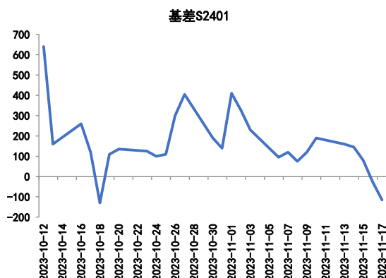
图3：工业硅期货合约S2401基差
