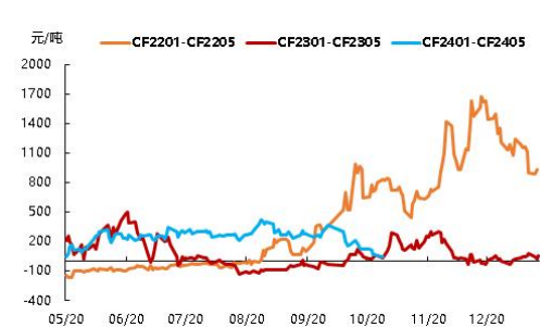
图 3：1-5 价差
