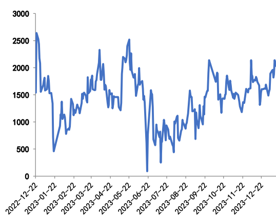
图5：工业硅4210基差
