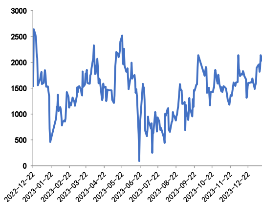
图5：工业硅4210基差
