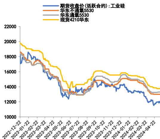
图3：工业硅不通氧5530基差
