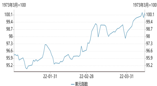
图 6：美元指数
