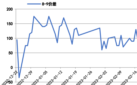
图6：8-9价差
