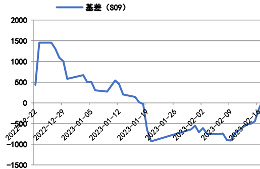
图4：基差（S09）
