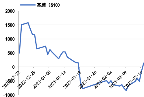
图5：基差（SI10）
