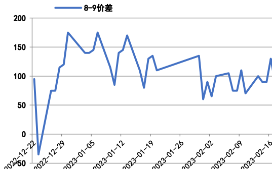
图6：8-9价差
