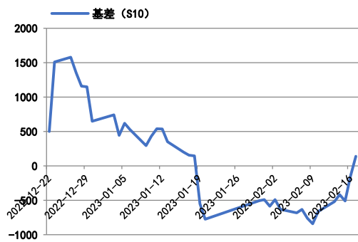
图5：基差（S10）
