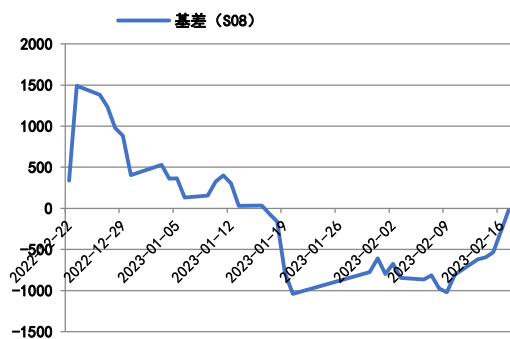
图3：基差（S08）
