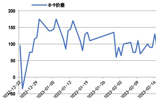
图6：8-9价差
