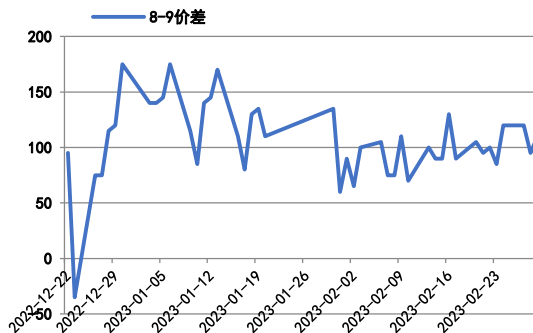
图6: 8-9价差
