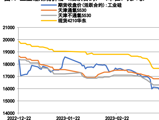
图1：工业硅期现价（活跃合约）（单位：元/吨）
