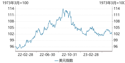
图 6：美元指数
