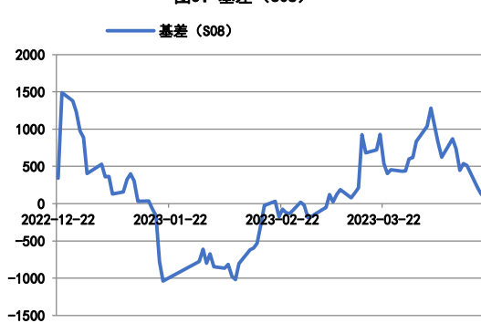
图3：基差（S08）
