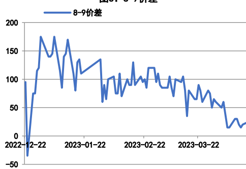
图6：8-9价差
