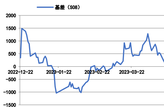
图3：基差（S08）
