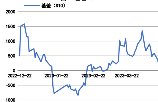
图5：基差（S12）
