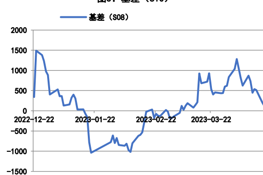
图3：基差（S10）
