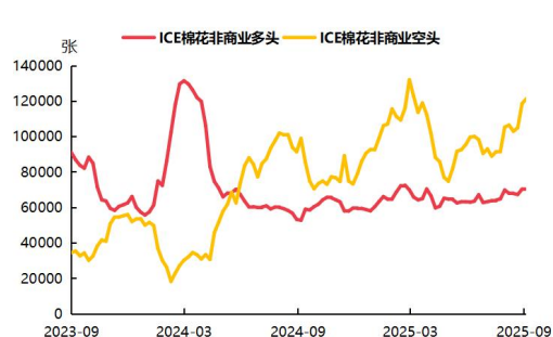
图 8：非商业持仓
