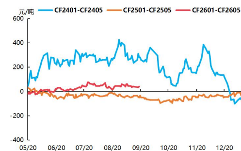
图 3：1-5 价差
