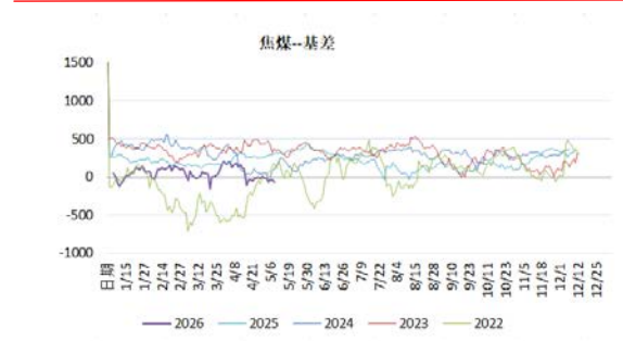
图 7：焦煤基差
