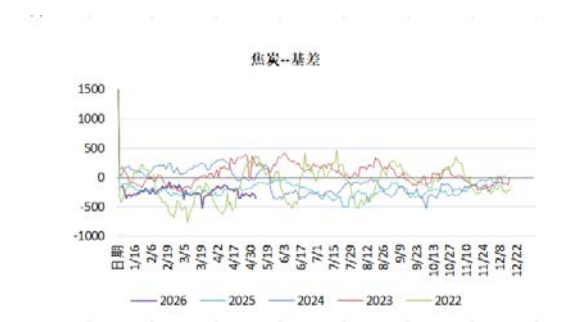
图 9：焦炭基差
