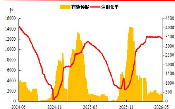
图 7：仓单数量
