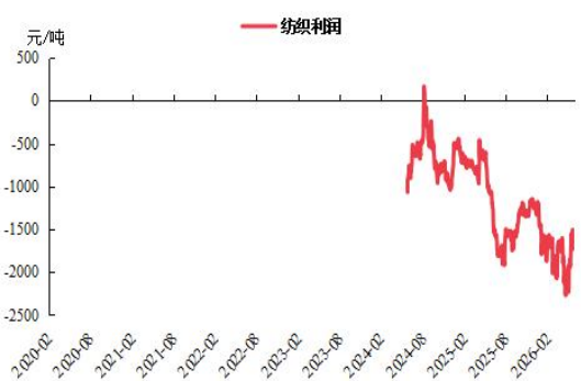
图 4：纺织利润
