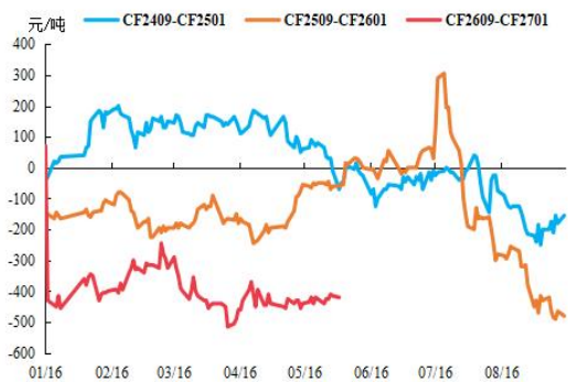
图 3：9-1 价差
