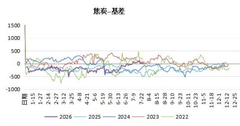
图 9: 焦炭基差
