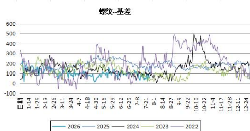
图 1：螺纹钢基差
