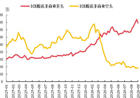
图 8：非商业持仓
