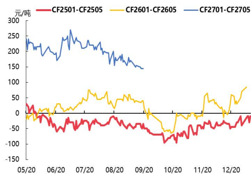
图 3：1-5 价差
