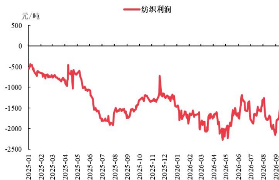
图 4：纺织利润
