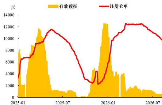
图 7：仓单数量
